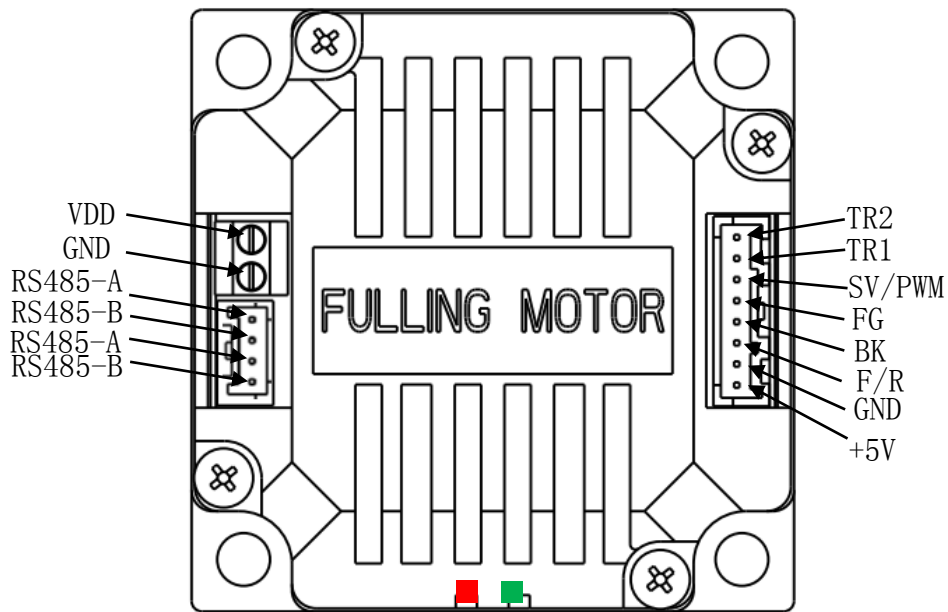
图 2 端子定义图
