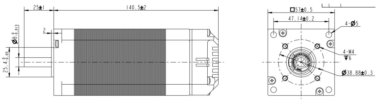
图 1 机械尺寸图
