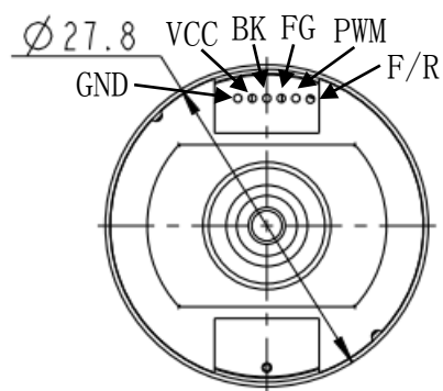
图2 引出线定义图
