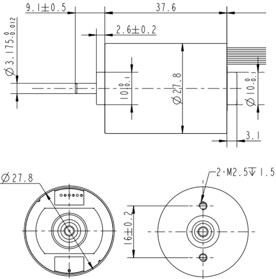
图1 机械尺寸图
